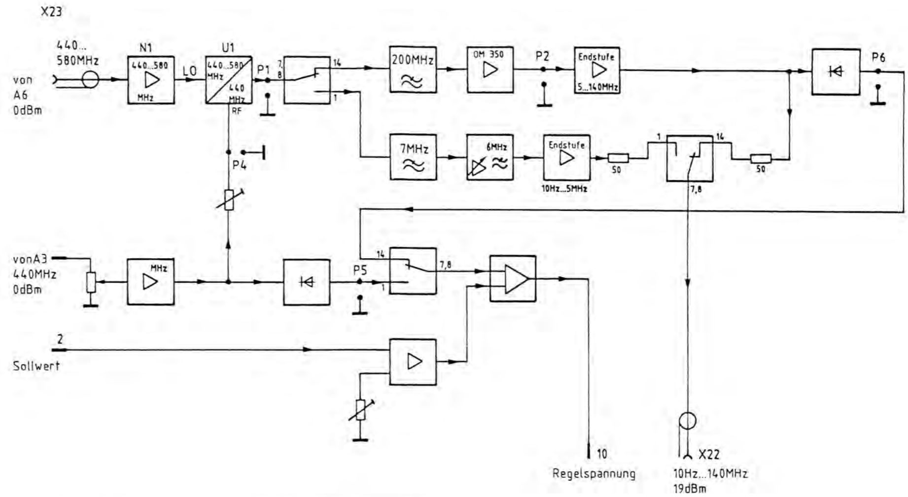
Bild 5-1 Blockschaltbild Ausgangsstufe
